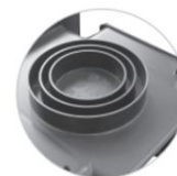
Scarico inferiore: \phi 75 - 90 - 110 e 80 - 100 - 125
